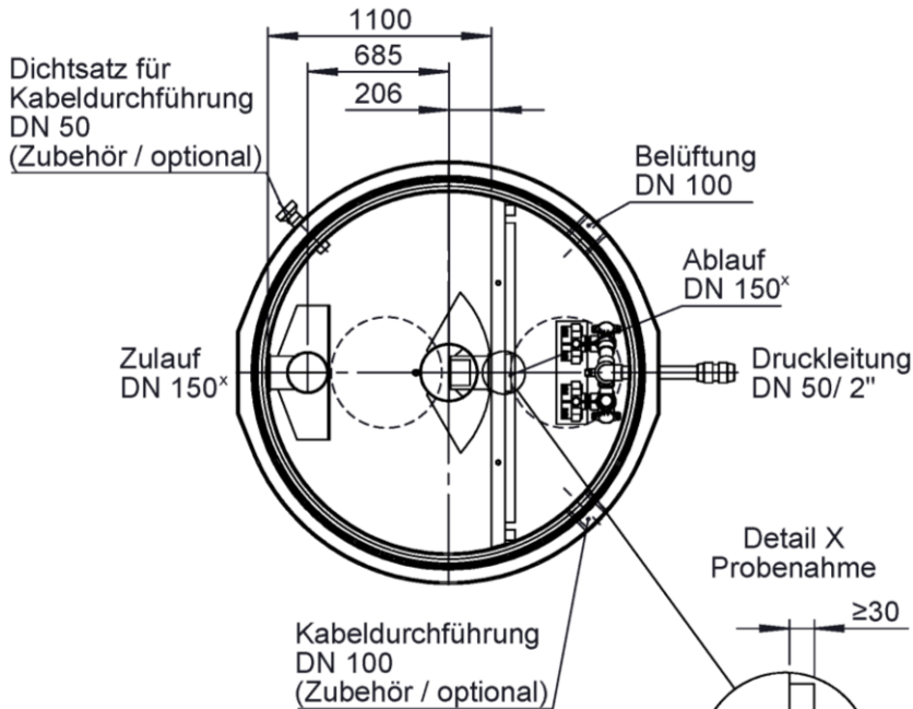
Ansicht Y
