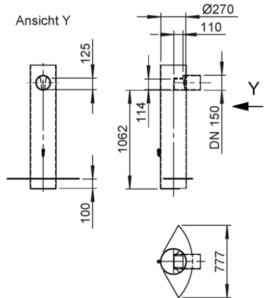
Abscheiderauslauf
