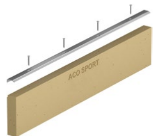
Klemmstein mit Klemmschiene
