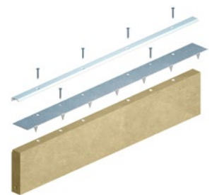
Einfassungsbord mit Krallschiene für Shockpad Dränageplatten und Klemmschiene für Kunstrasen
