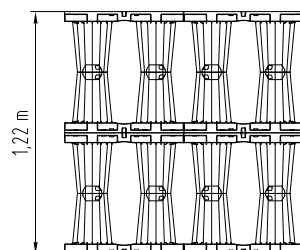
ACO Stormbrixx HD zwei Lagen
