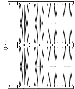
ACO Stormbrixx SD zwei Lagen
