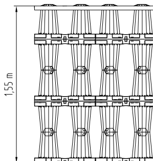
ACO Stormbrixx HD zweieinhalb Lagen
