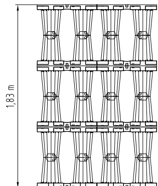
ACO Stormbrixx HD drei Lagen
