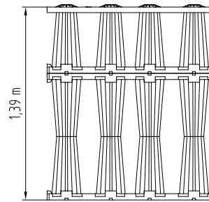
ACO Stormbrixx SD eineinhalb Lagen
