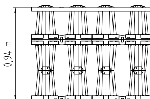
ACO Stormbrixx HD eineinhalb Lagen
