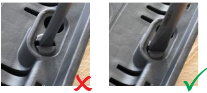
Jetzt wird die Profiline X auf die Verstelleinheit gestellt und von oben eingedrückt bis die Verstelleinheit hörbar einrastet. Nun ist die Höhenverstellung voll funktionsfähig.
