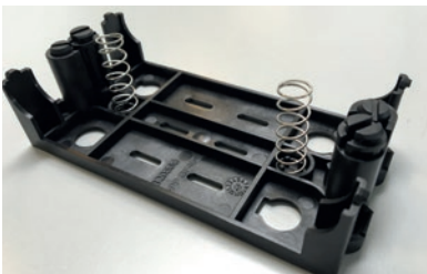
Komplette Verstelleinheit ACHTUNG: Nicht verändern
