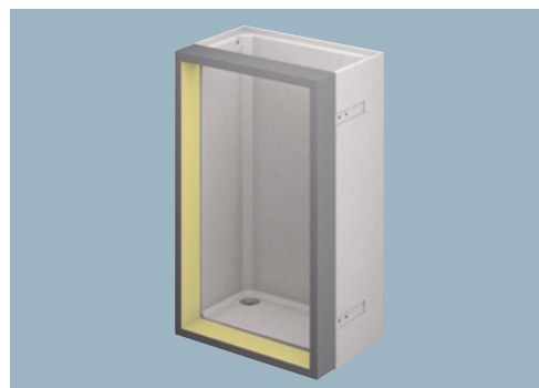
Betonlichtschacht in druckwasserdichter Ausführung mit umlaufend aufgebracht er Dämmrahmen zum Aufstapeln eines weiteren Schachtes mit angeschraubter Hinterfüllplatte
