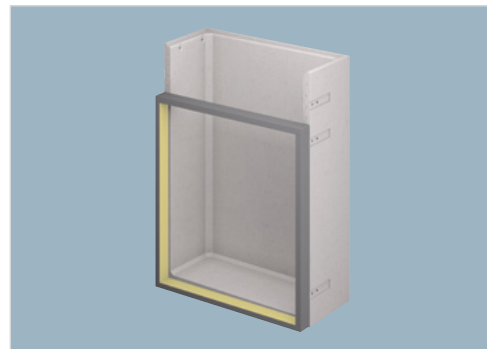
Betonlichtschacht in druckwasserdichter Ausführung mit umlaufend aufgebracht er Dämmrahmen zum Aufstellen einer Hinterfüllplatte und zusätzlichem Befestigungsbereich zur Verschraubung der Hinterfüllplatte mit dem Schacht
