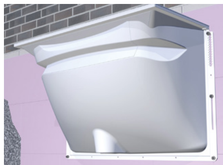
Montagebeispiel Art.-Nr. 380420 bis 380425
