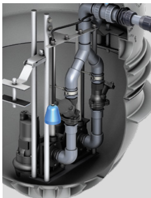
Die ACO Pumpstation Powerlift-PSD-PE zeichnet sich durch eine besonders kompakte Bauweise aus
