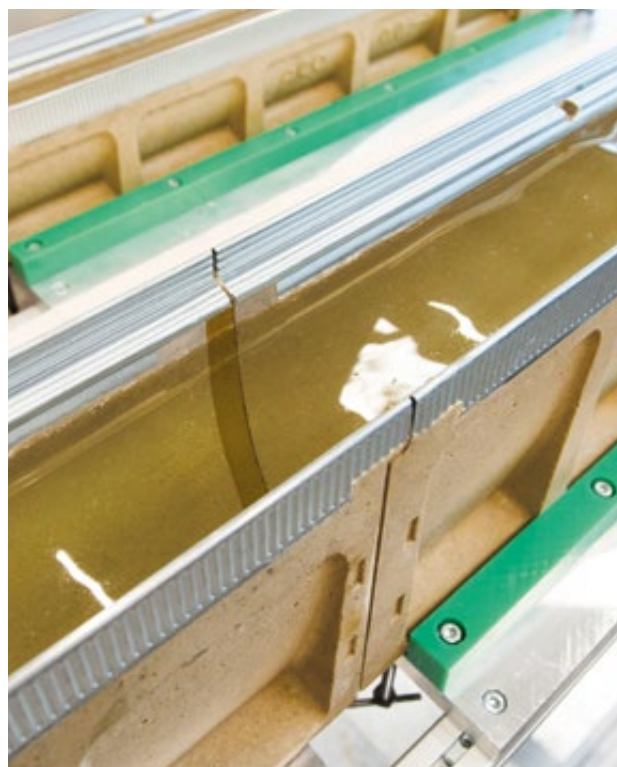
Prüfung der Dichtheit
