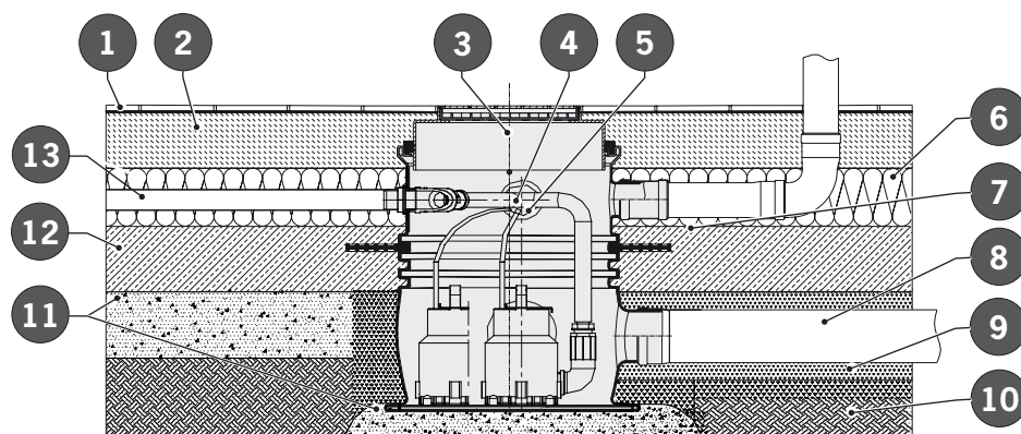
Abb.: Bodenaufbau ohne Dämmung
