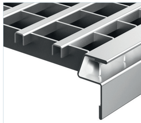
Designrost Längsprofil, Edelstahl oder Stahl verzinkt, begebar bis 1,5 kN
